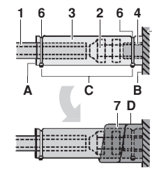
Трубопровод жидкого хладагента
