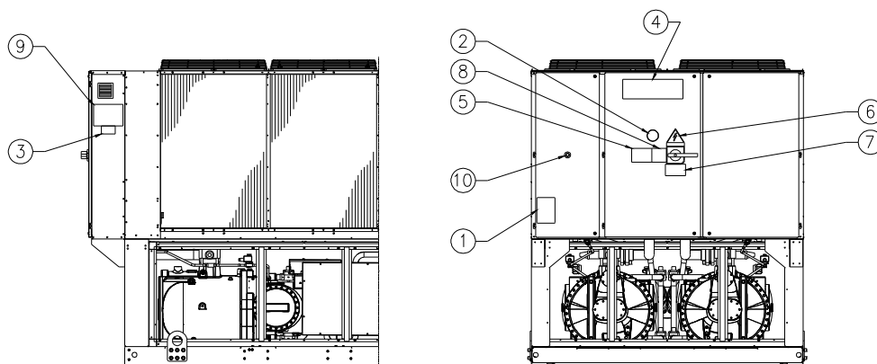
Obrázok 1 – Popis štítkov aplikovaných na elektrickom paneli (Elektrický panel môže byť z dvoch rôznych výšok)
