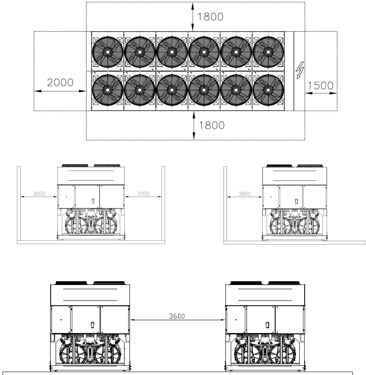
Kuva 4 - Tilan minimivaatimukset
