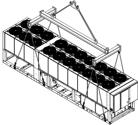
Kuva 3 - Yksikön nostaminen
