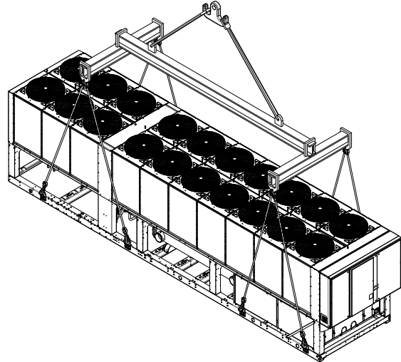
Slika 3 - Podizanje jedinica
