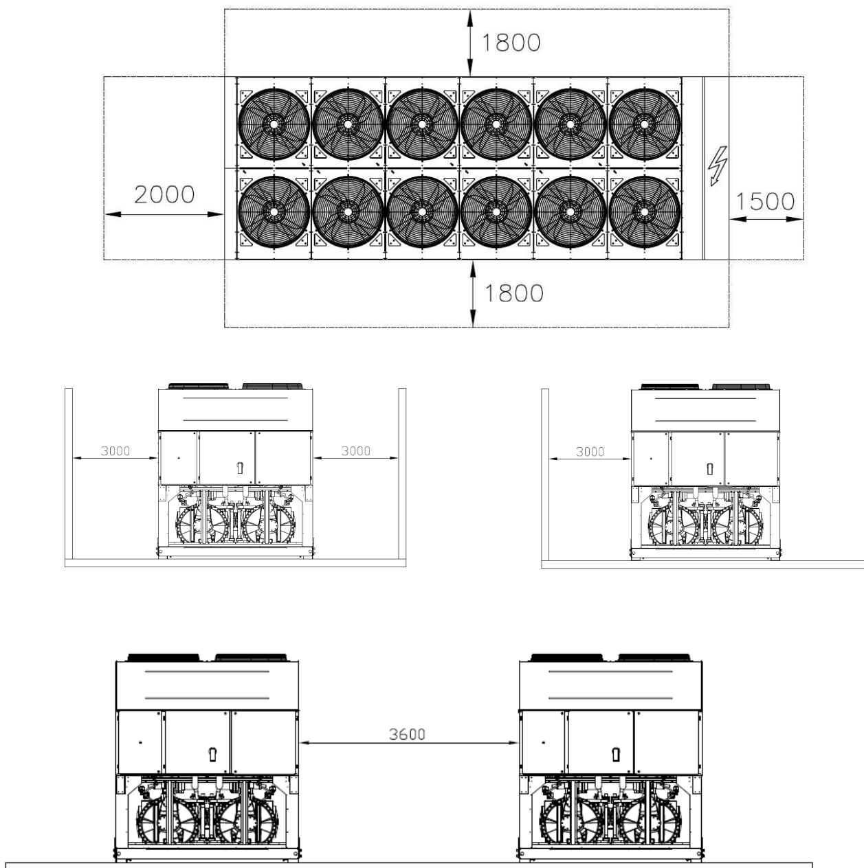
Abbildung 4 – Mindestabstände
