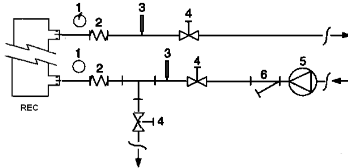
Kuva 6 - Vesiputkien liitännät lämmöntalteenottoon tarkoitetuilla lämmönvaihtimilla
