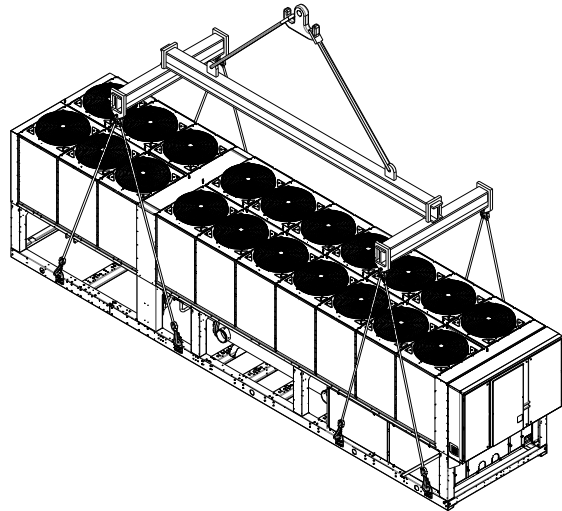
háromkompresszoros egység
