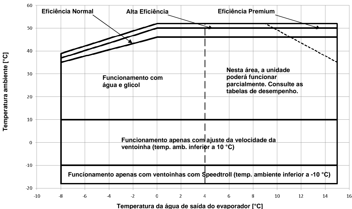
Figura 2 – Limites operativos
