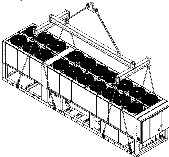
Рисунок 3 – Подъем агрегата
