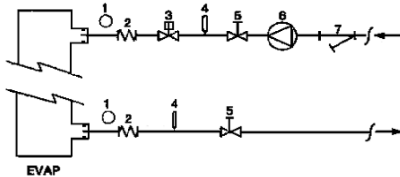
Kuva 5 - Vesiputkien liitännät höyrytimeen
