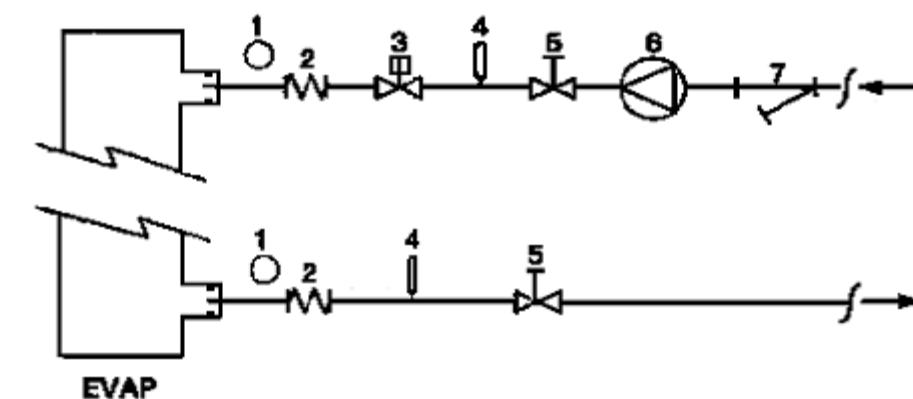
Rysunek 5 – Podłączenie rur wodnych do parownika
