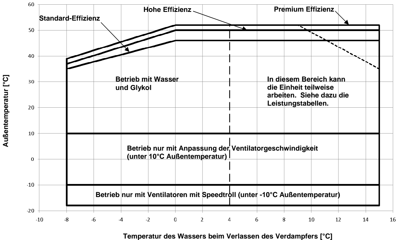
Abbildung 2 - Betriebsbereich
