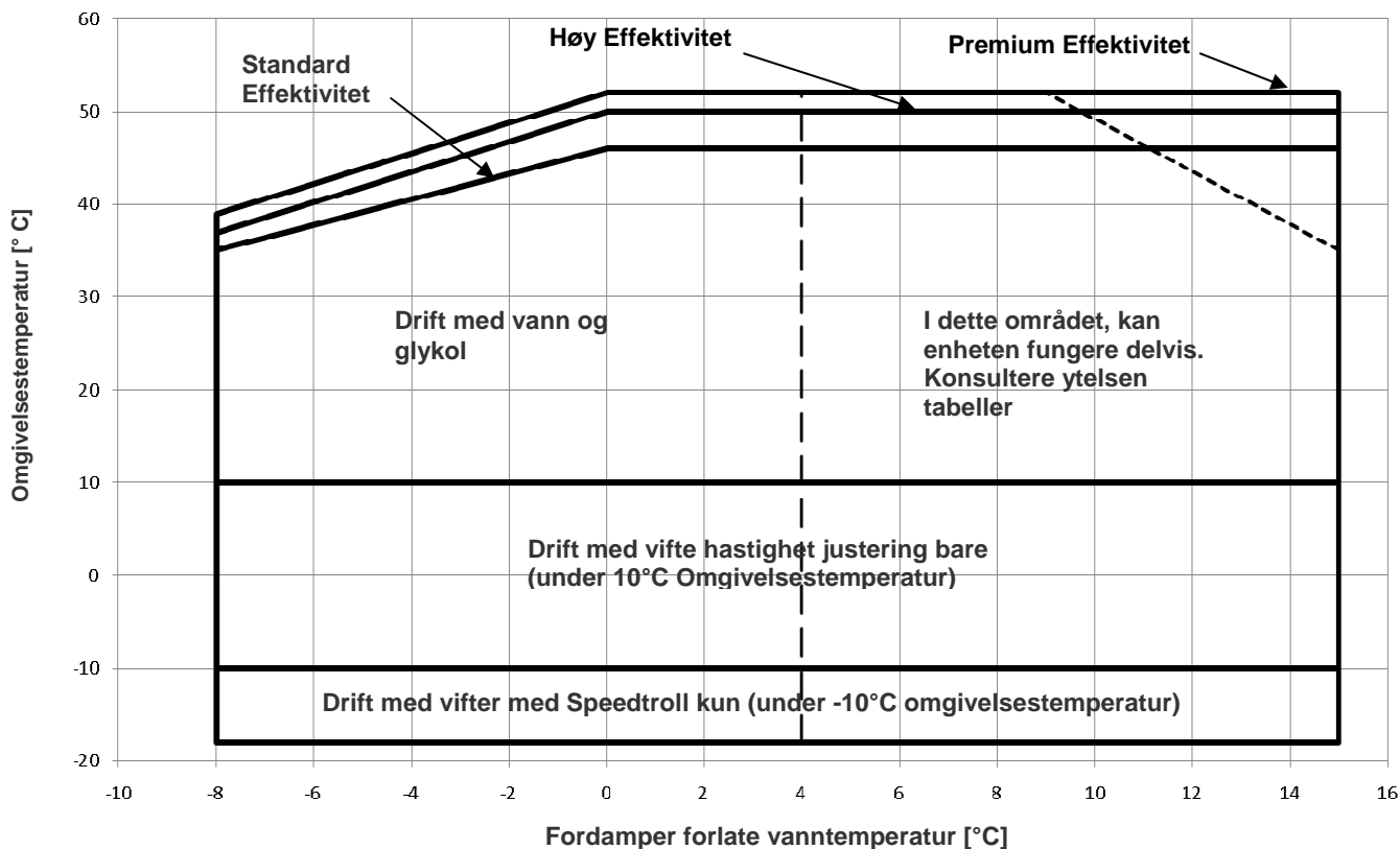
Figur 2 - Belastningskapasitet
