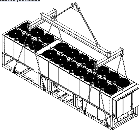
3 jednostki sprężarki
