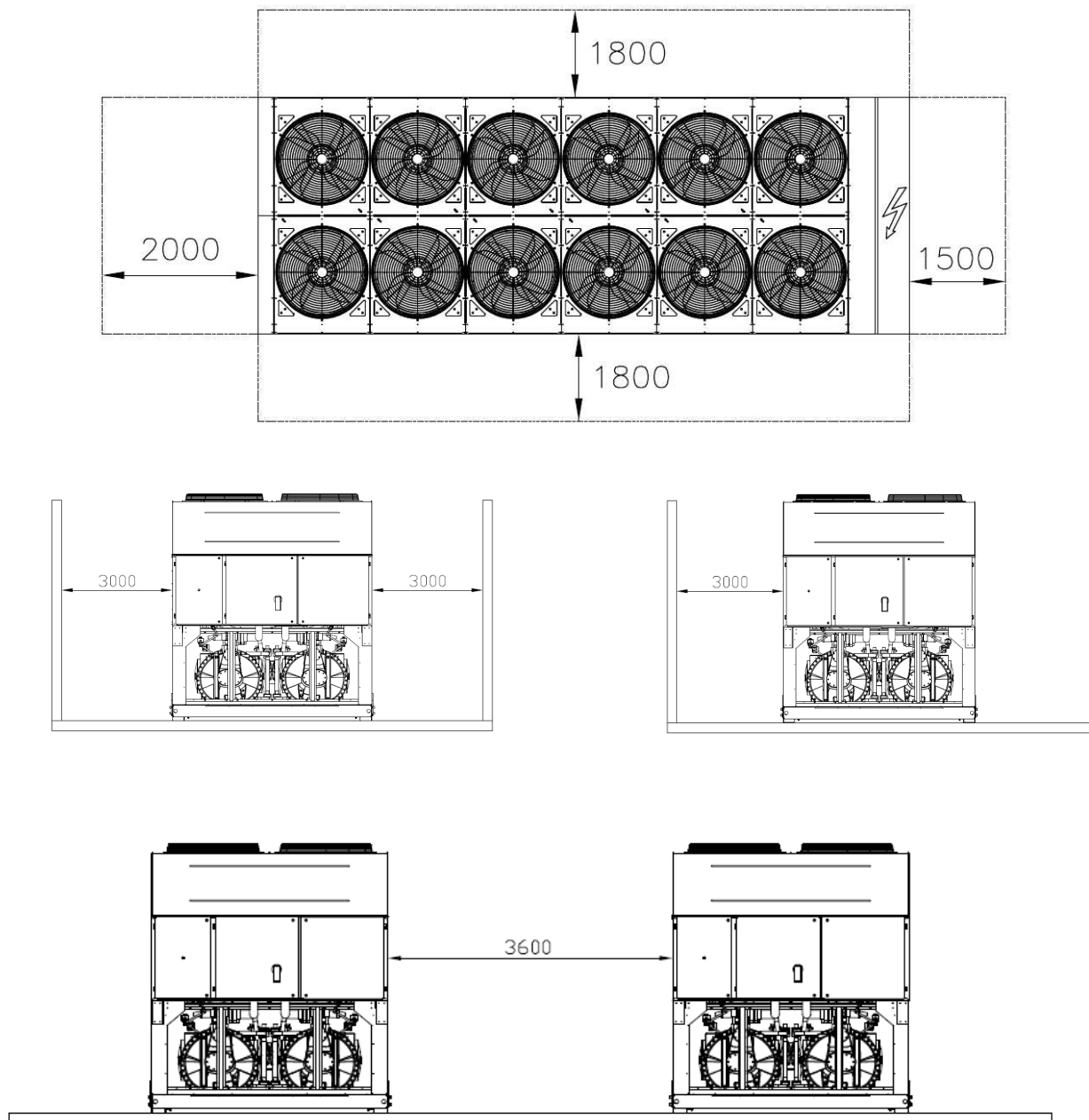
Figur 4 – Minsta platskrav
