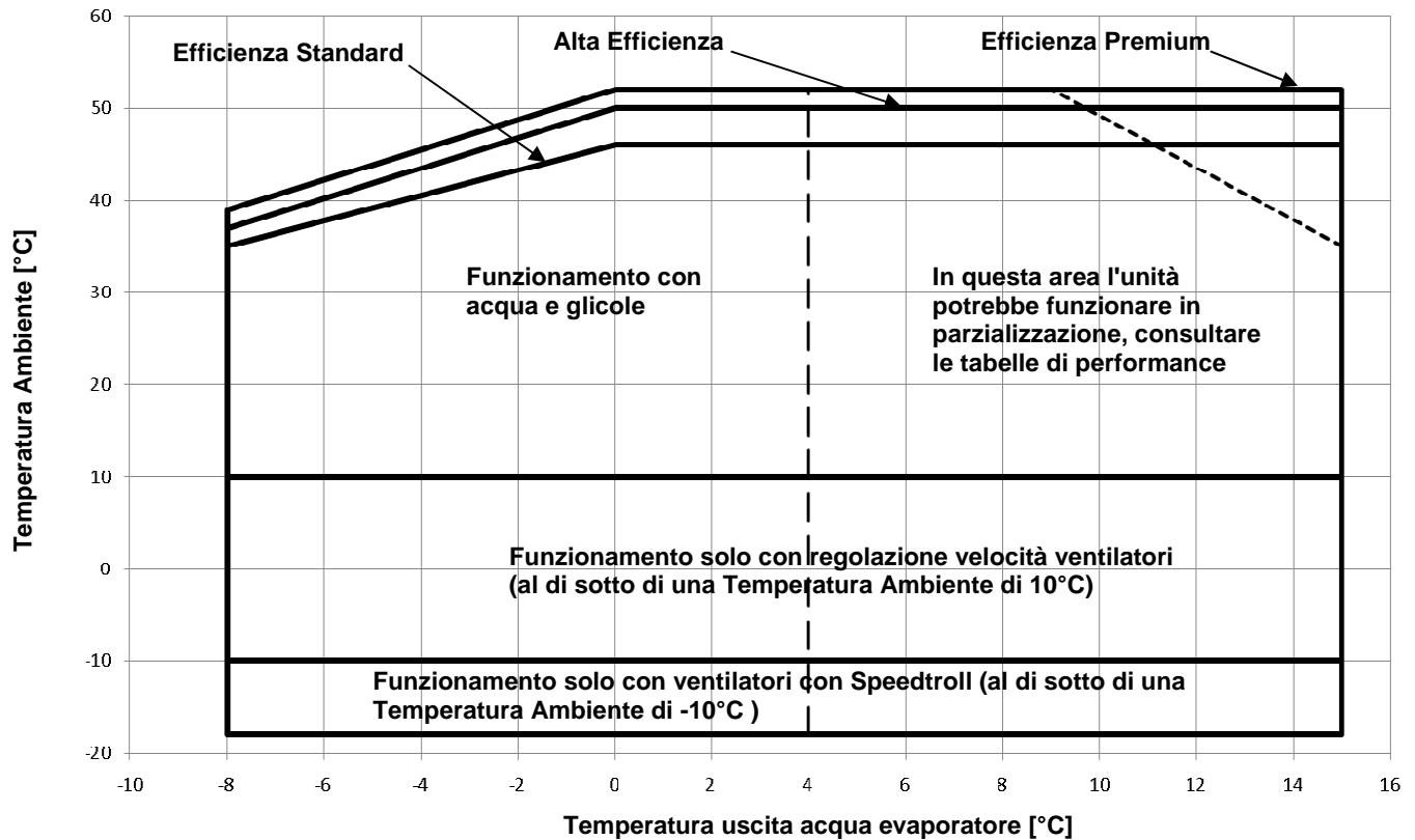
Figura 2 – Limiti operativi
