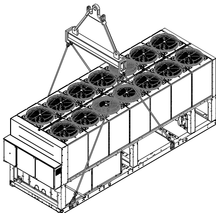
Rysunek 3 - Podnoszenie jednostki
