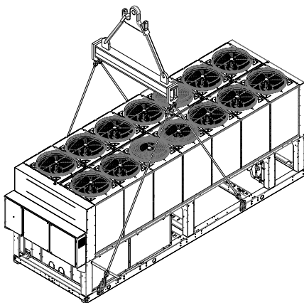
eenheid met 2 compressors
