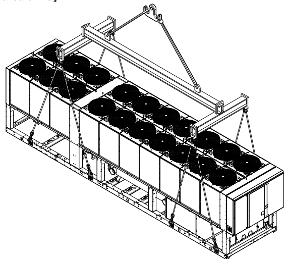
Figura 3 – Ridicarea unității
