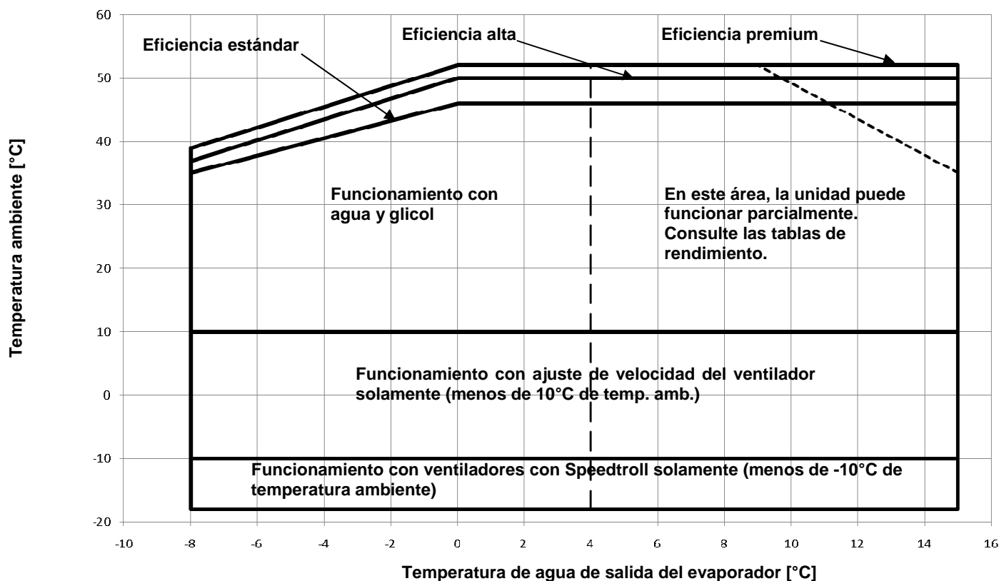
Figura 2 - Límites operativos
