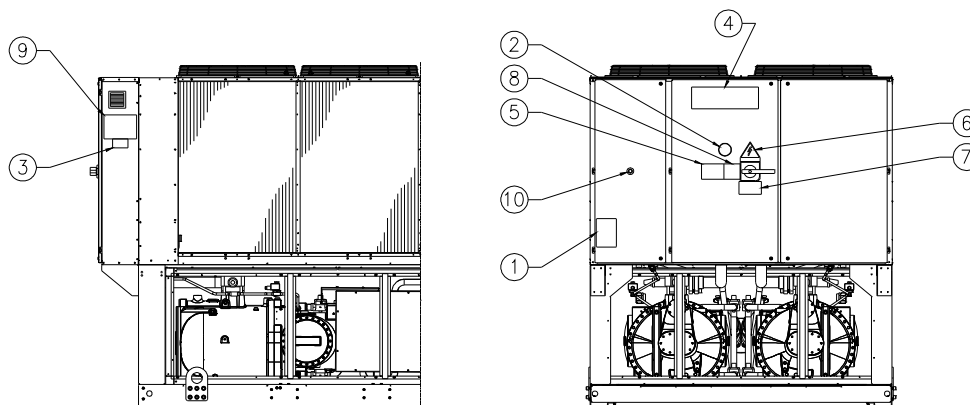
Схема 1 – Описание на етикетите поставени на електронният пулт (Електрическо табло може да бъде на две различни височини)
