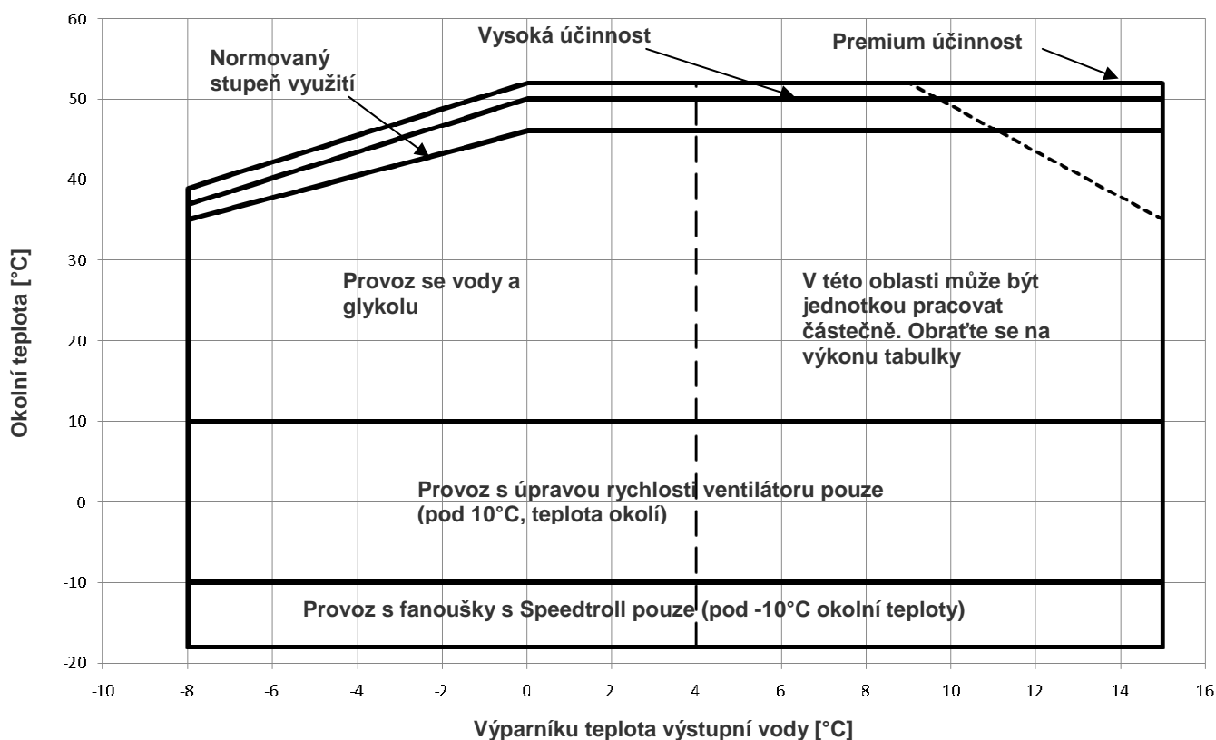
Obrázek 2 - Provozní limity
