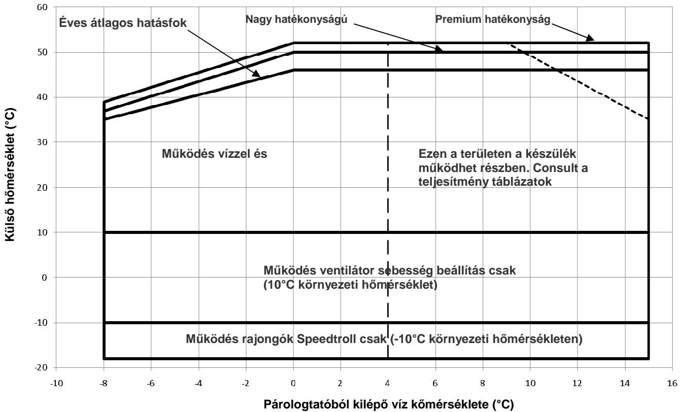
Ábra 2 – Üzemi tartomány
