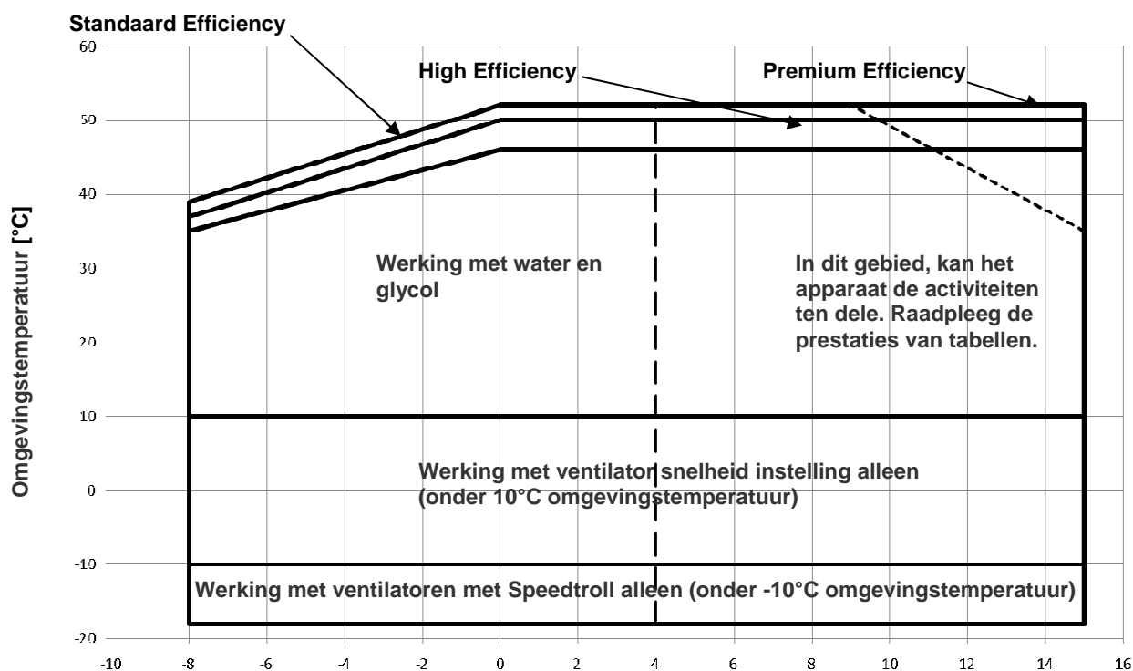
Figuur 2 – Werkingslimieten
