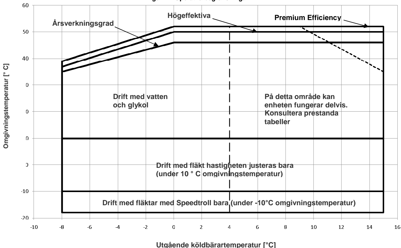
Figur 2 – Operatva begränsningar
